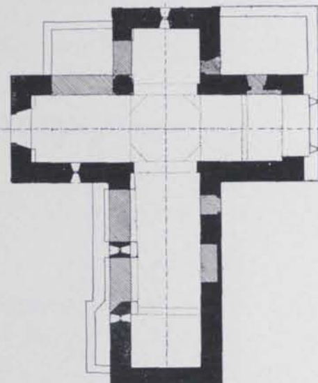
Fig. 335. — Planta de l'església de Santa Maria, de Castellfullit de Riubregós
